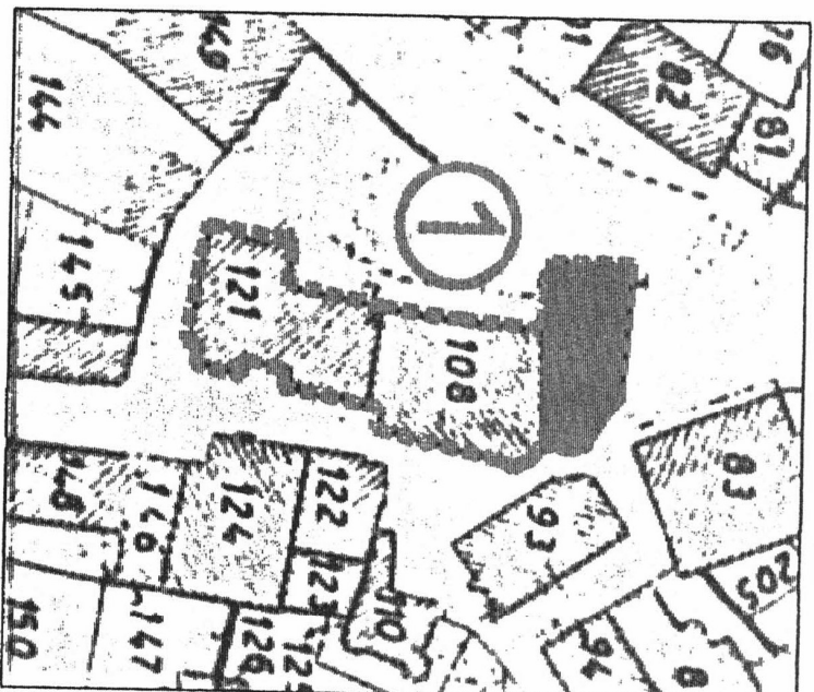
QUADRONI- CENTRO STORICO ISOLATO 1 - VIA DELLA PARCELLA FOGLIO N. 6 - PARTICELLA N. 92
